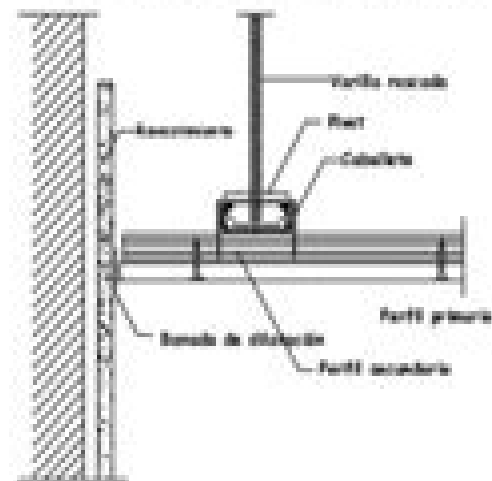
Encuentro con revestimiento
