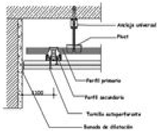
Encuentro con pared
