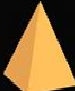
pyramid
