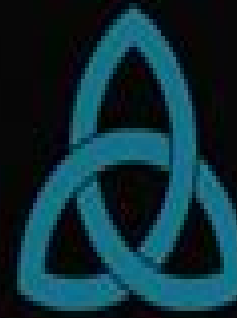
triquetra
