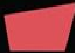
trapezium
