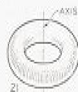
21 TORUS
