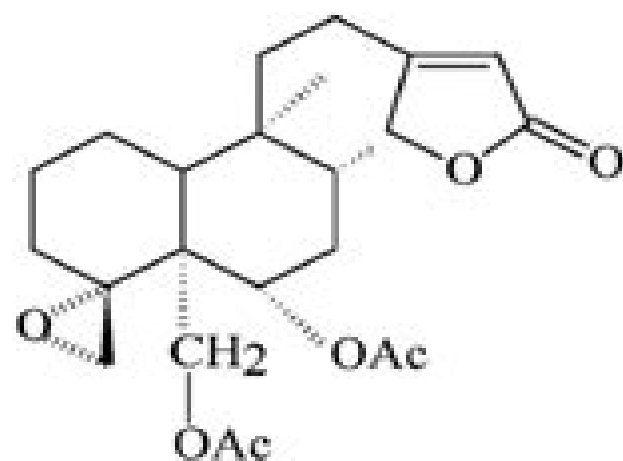
Ajugarin I
