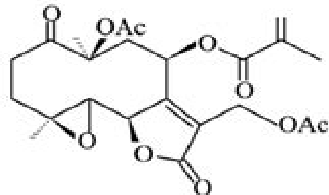
Glaucolide-A
