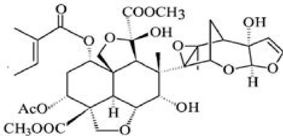
Azadirachtin
