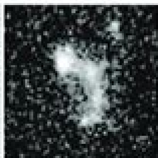
bent chains (1.01)
