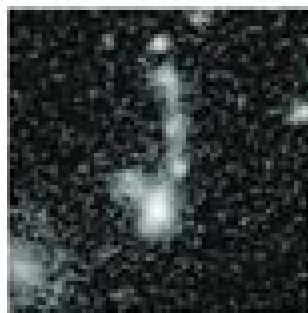
bent chains (1.01)
